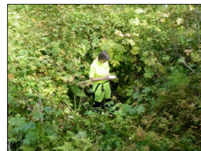
En fångstgrop i Ullådalen, Åre kom- mun, återbesökt. Gropen ingår i ett system om fem fångstgropar med avsevärda djup, ned mot 2 meter och troligen använda långt fram i tiden.
